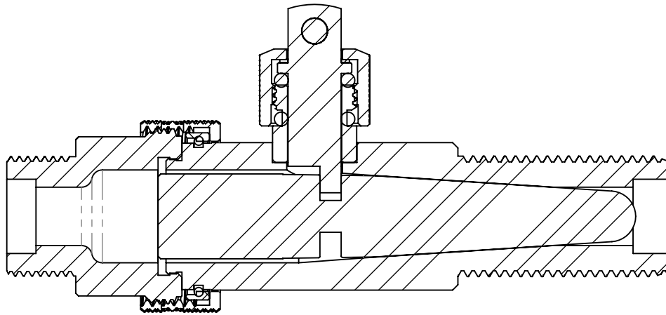
A-A (1 : 1)
