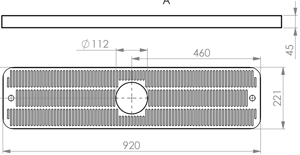
A-A (1 : 8)
